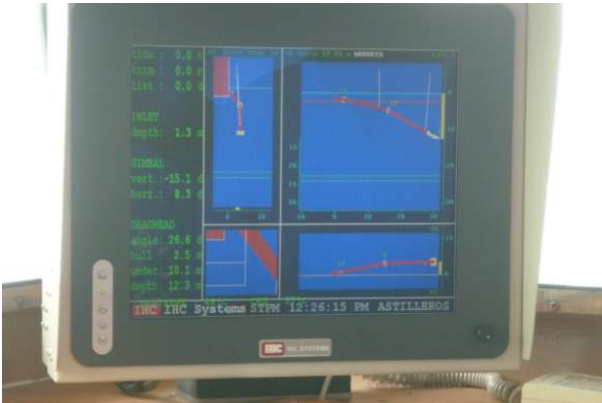
Fotografía 4. Equipo que monitorea el brazo hidráulico de la draga, durante las operaciones de succión del material del fondo marino, en el sector de la Boya 51, del Canal de Acceso al Puerto Marítimo de Guayaquil, Junio del 2010.
